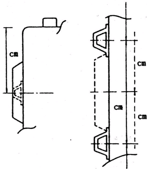
防舷材測定位置図
