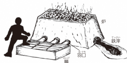
箱形製鉄炉の解説イラスト
