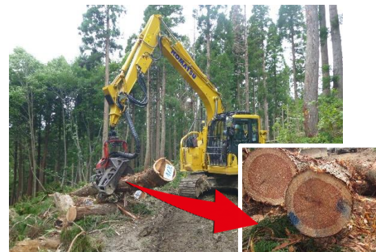
マーキング機能を備えたハーベスタで仕分け作業等の効率化を実証
