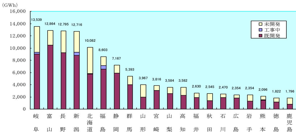
図 都道府県別包蔵水力（上位20都道府県）
