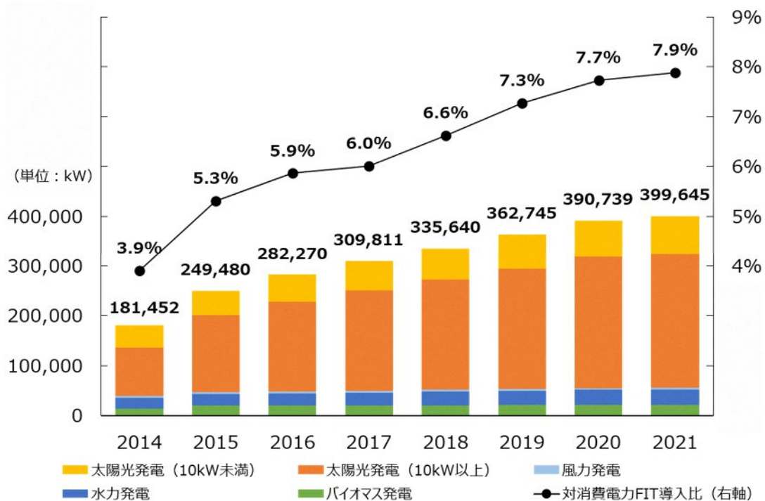
図 2-52 県内の FIT 導入容量の推移
