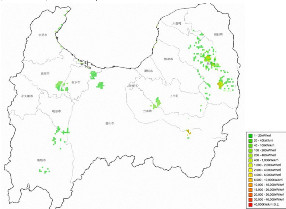
11 図 2-58 地熱発電（蒸気フラッシュ・バイナリー・低温バイナリーの合算）の導入ポテンシャルの分布図
