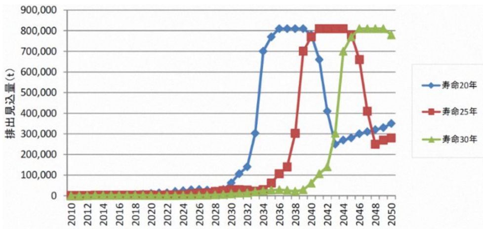
12 図 2-24 太陽光パネルの排出見込
