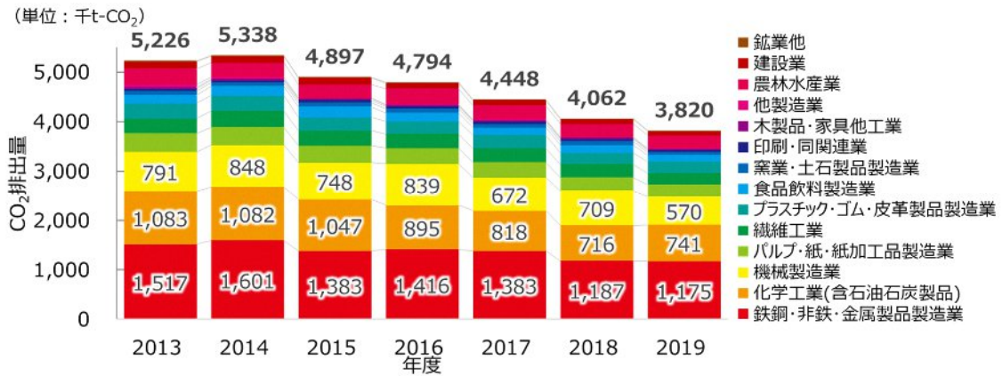
7 図 2-33 富山県の産業部門の業種別 CO 2 排出量の推移
