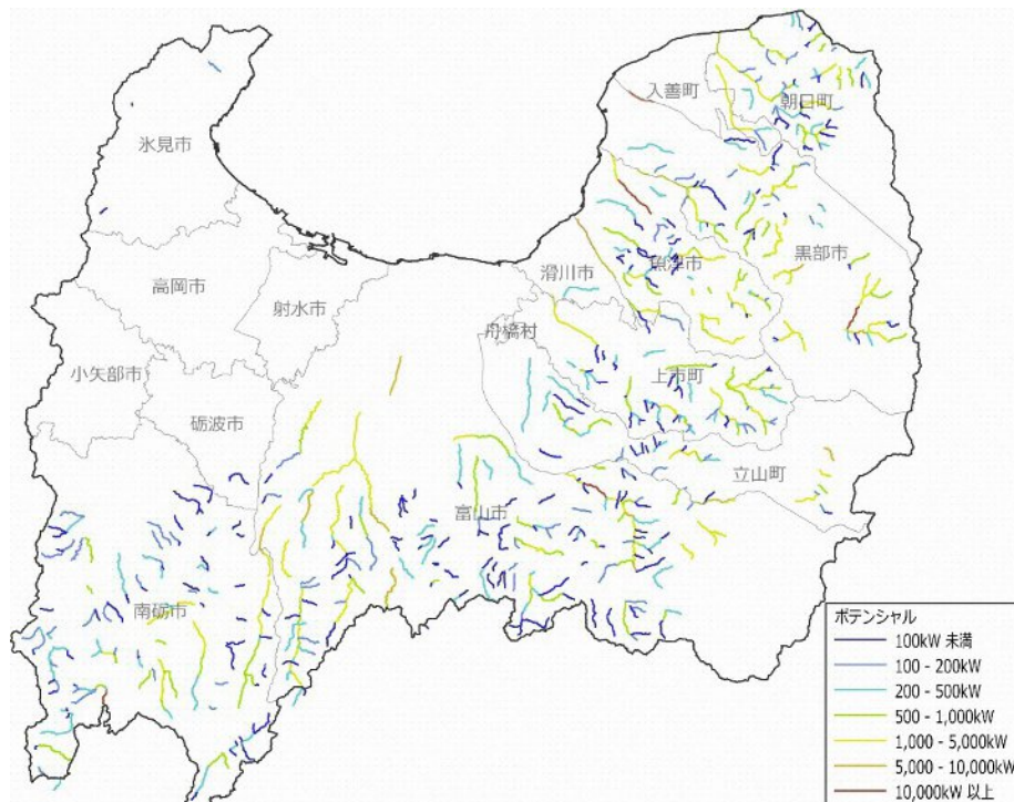
10 11 図 2-56 中小水力発電（河川）の導入ポテンシャルの分布図
