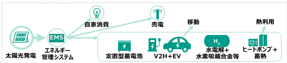
33 図 6-3 太陽光発電設備とエネルギー管理システム、エネルギー貯蔵設備等の併用
