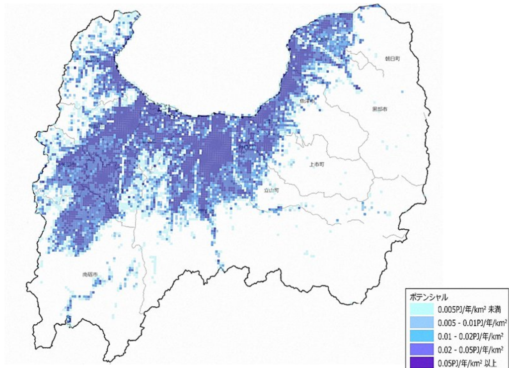
図 2-60 地中熱利用の導入ポテンシャルの分布図
