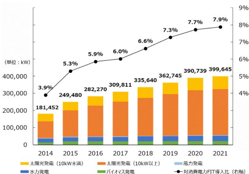
富山県内の FIT 導入容量の推移 (再掲：図 2-52)
