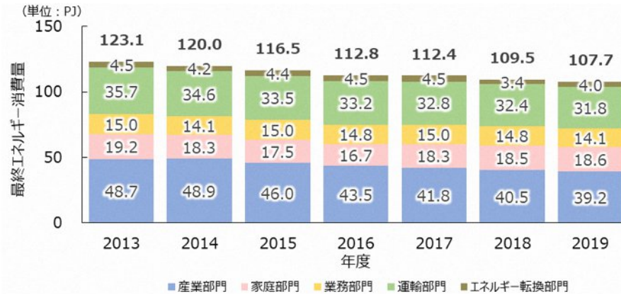
6 図 2-43 富山県の最終エネルギー消費量の推移
