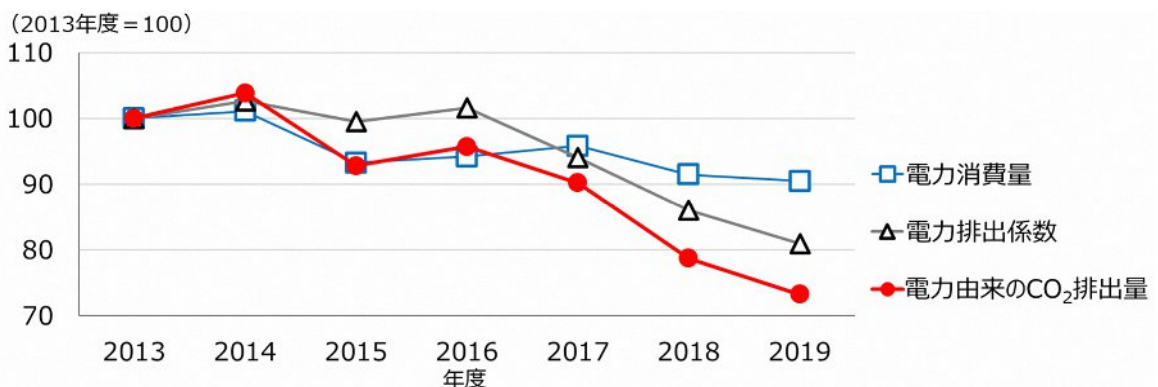
12 図 2-35 富山県の産業部門の電力からのCO 2 排出量と電力消費量、電力排出係数の推移
