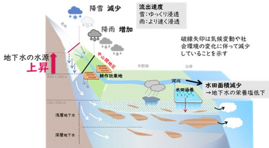
図 7-24 水・栄養塩循環の模式図
