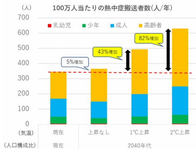
図 7-36 年齢層別の熱中症搬送者数の将来予測
