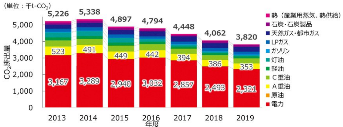
4 図 2-34 富山県の産業部門の燃料別 CO 2 排出量の推移
