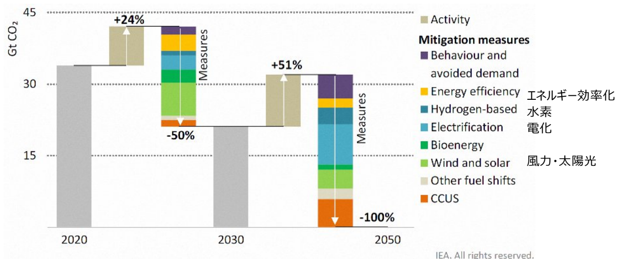
16 図 2-5 CO 2 排出ネットゼロシナリオにおける排出削減
