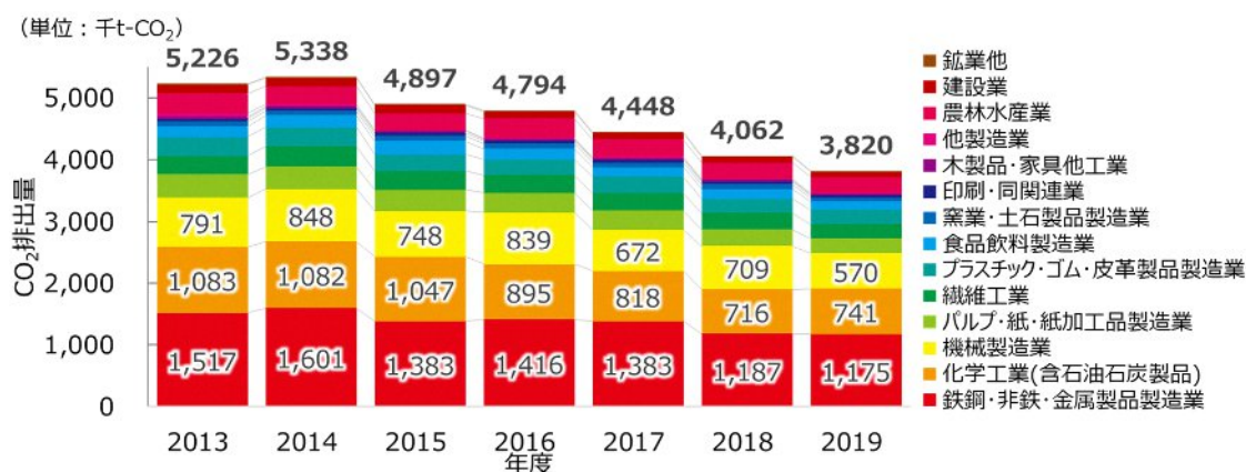
7 図 2-33 富山県の産業部門の業種別 CO 2 排出量の推移
