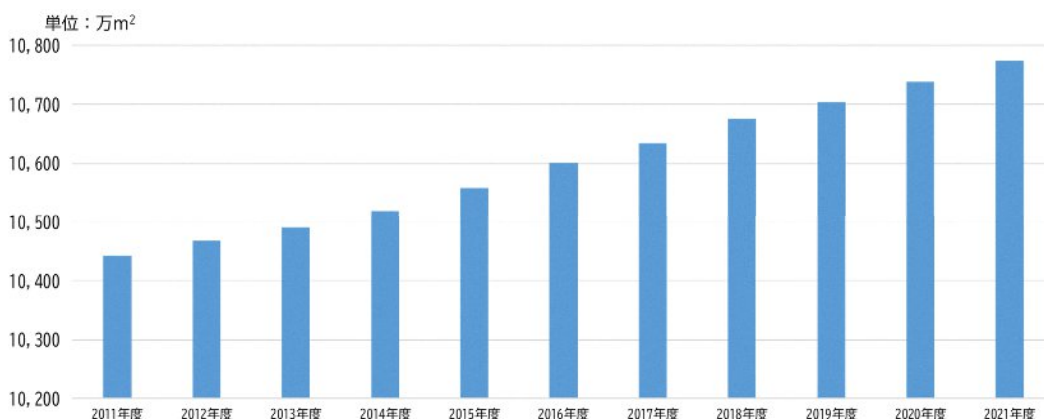
21 図 2-30 富山県内の建物用途別延床面積の推移
