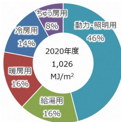
28 図4-3 業務他部門の用途別エネルギー消費原単位
