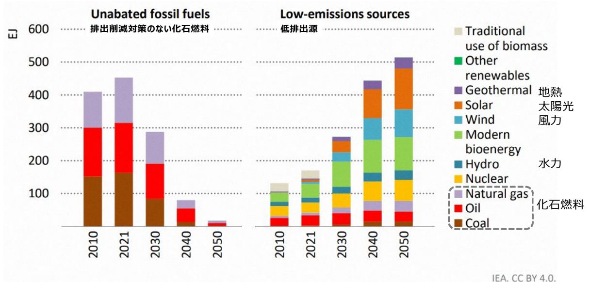
8 図 2-4 CO 2 排出ネットゼロシナリオにおける一次エネルギー供給の構成
