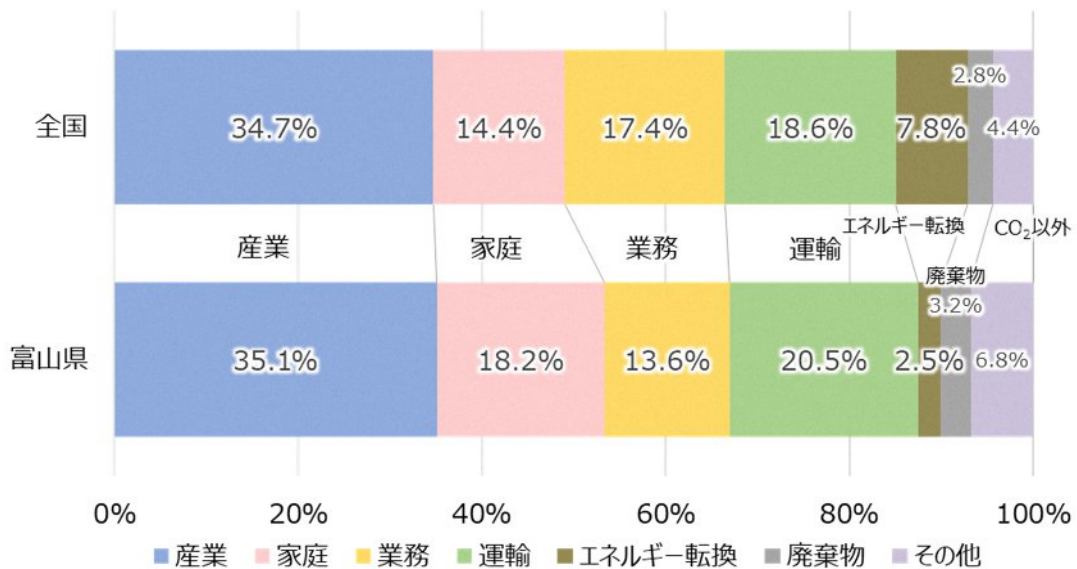
5 6 図 2-32 富山県と全国の温室効果ガス排出量（2019 年度）の内訳
