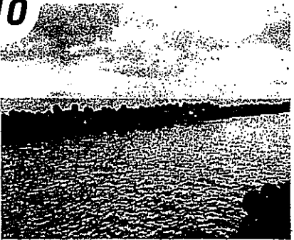
滑川海岸海岸保全異形 ブロック据付工(三穂地内)
