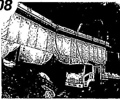
砂防関係施設整備(急傾斜) 崩壊土砂防止柵工(本江地内)
