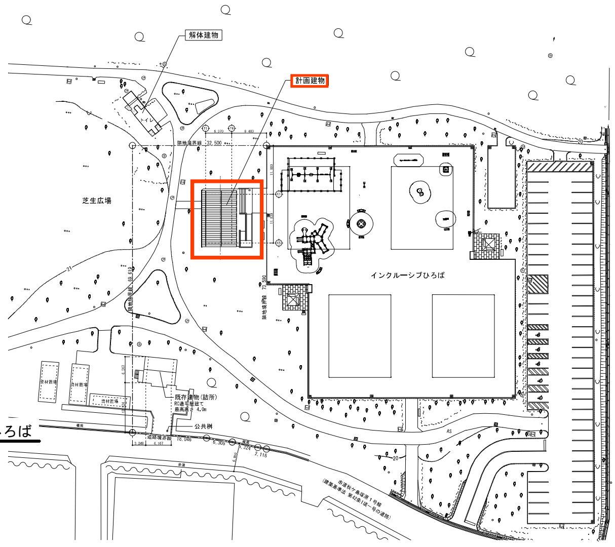
全体配置図 A1 S=1:300 A3 S=1:600
