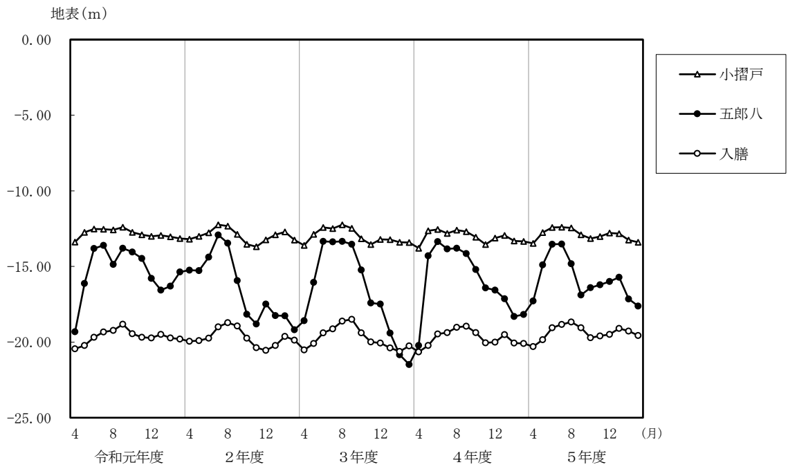
図 10-4 地下水位 (月平均値) の推移
