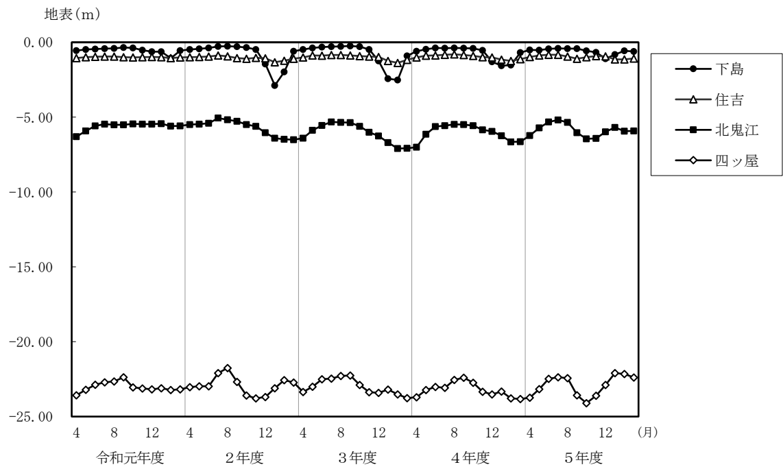
図 10-3 地下水位（月平均値）の推移
