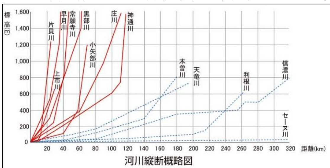
図4 河川縦断図
