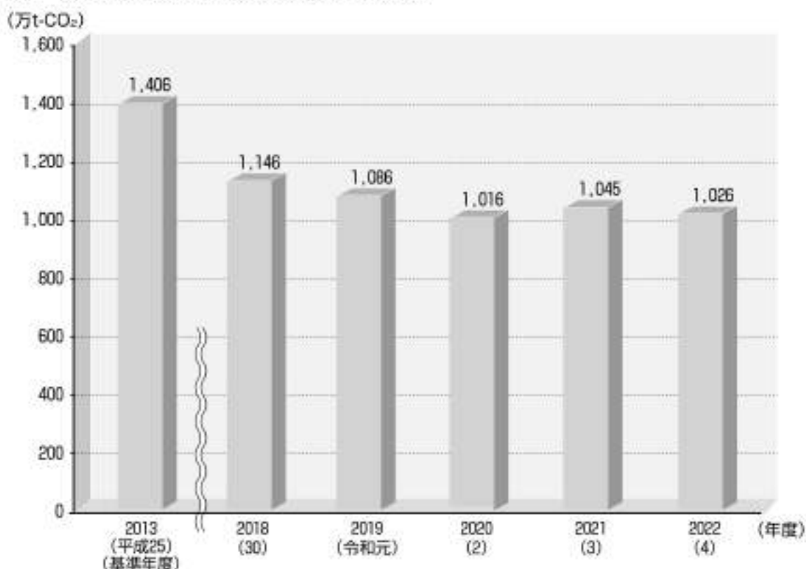
図2 県内における温室効果ガス排出量の推移
