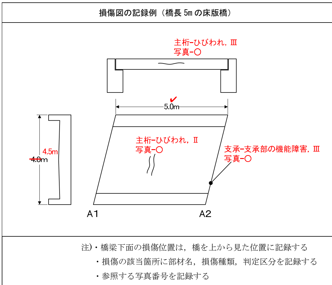
図 5.2 損傷図の記入例
