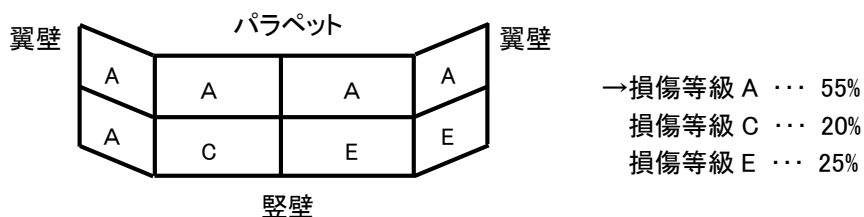
図 8.3 損傷等級の記録イメージ(橋台)
