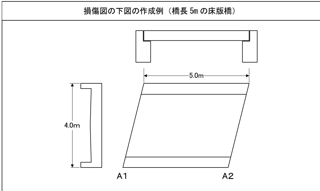
図 5.1 損傷図の下図例
