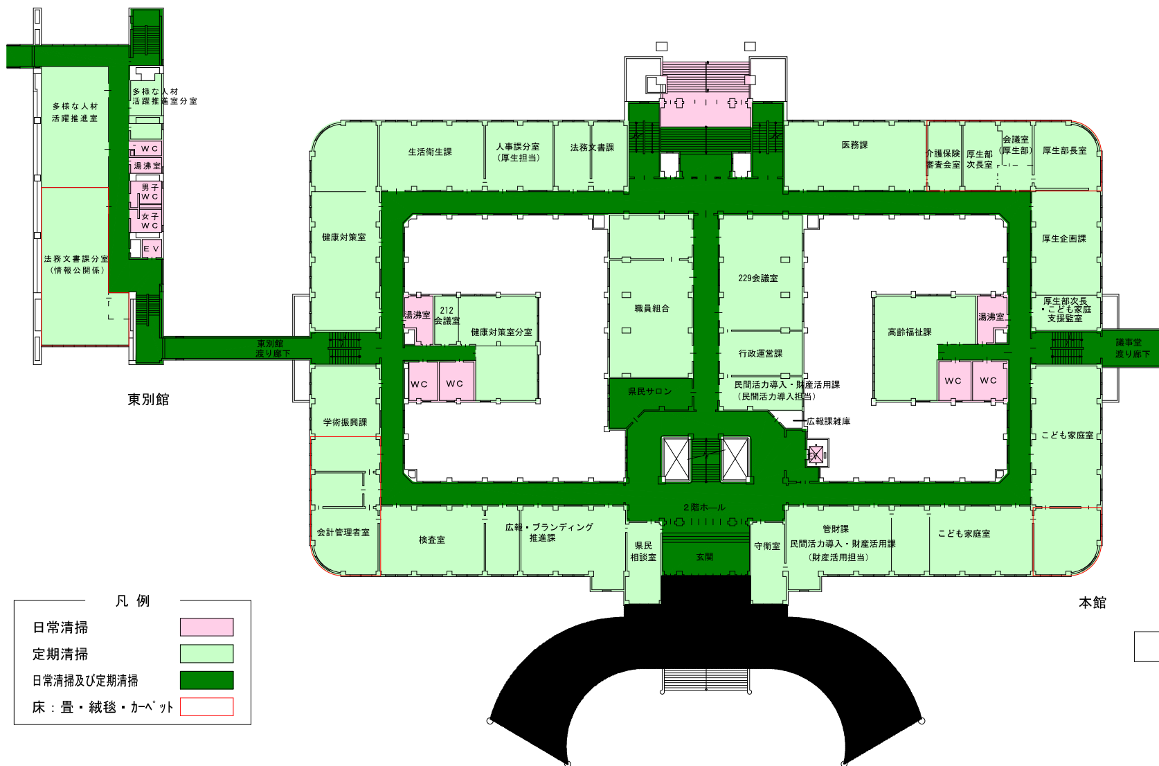
2 階平面図
