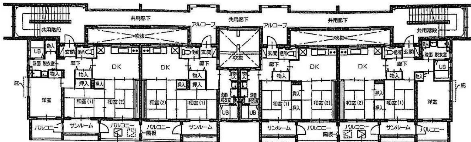
1~3階平面図
