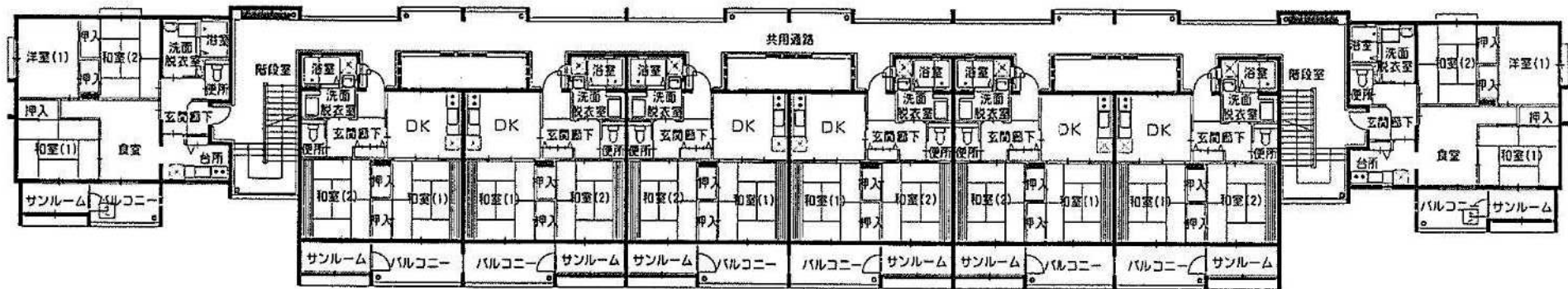
1～3階平面図
