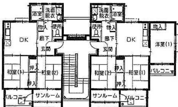
1~3階平面図
