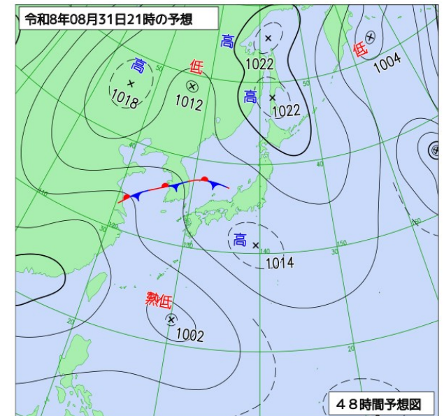
8月31日21時の予想天気図
