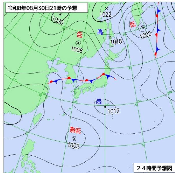
8月30日21時の予想天気図
