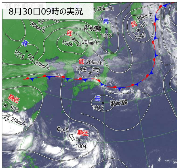
8月30日9時の 気象衛星ひまわり（赤外画像）を重ねた天気図
