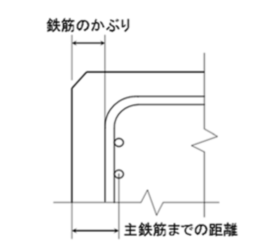
図 2-6-3 鉄筋のかぶり
