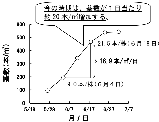
図10 茎数の推移 (生育観測ほ平年値) 注) H26~R5の平均
