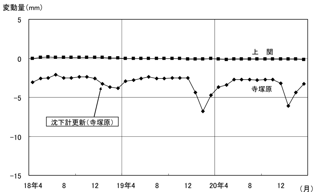
図13 地盤変動量の推移（月平均値）
