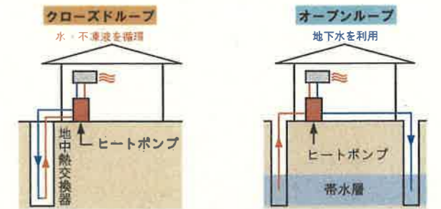
◇住宅・ビル等の冷暖房・給湯 ◇プール・温浴施設の加温 ◇農業施設の空調 ◇路面の融雪・凍結防止 地中熱ヒートポンプシステム (出典: 環境省)
